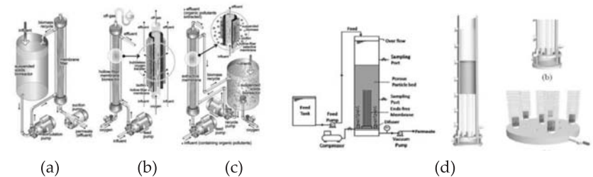
Gambar 2. Tipe bioreaktor membran: (a) MBR pemisahan biomassa, (b) MBR aerasi, (c) MBR ekstraktif, dan (d) MBR implanted ends-free (Wenten 2009)
