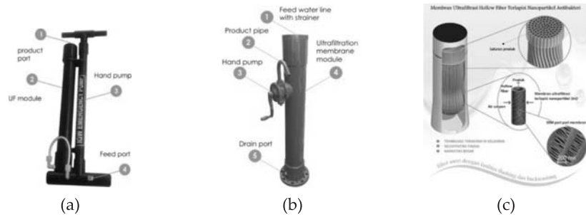
Gambar 1. Unit ultrafiltrasi untuk keperluan emergency: (a) UF emergency, (b) Green Ultrafilter, dan (c) semi industrial UF untuk aplikasi rumah tangga
