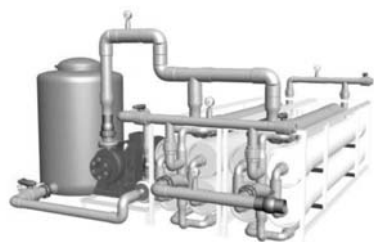
Gambar 3. Unit membran UF industri akuakultur
